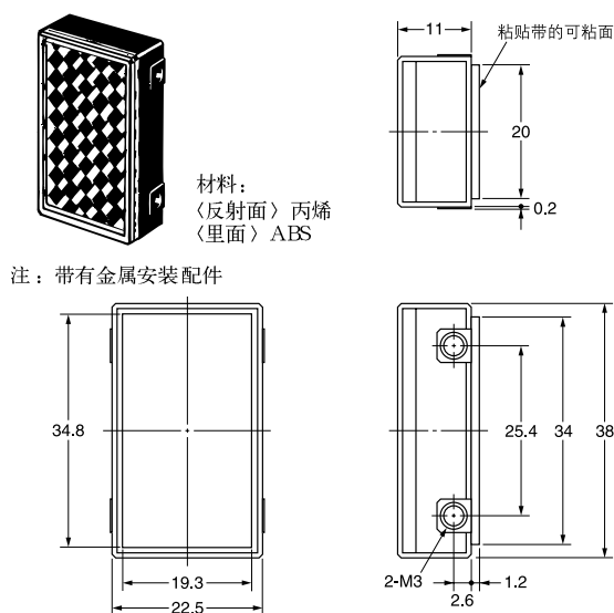
反射板(小型) 型号E39-R3
